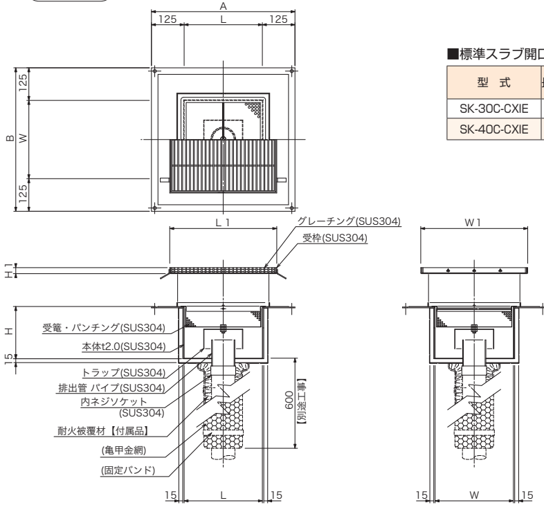
構造図
