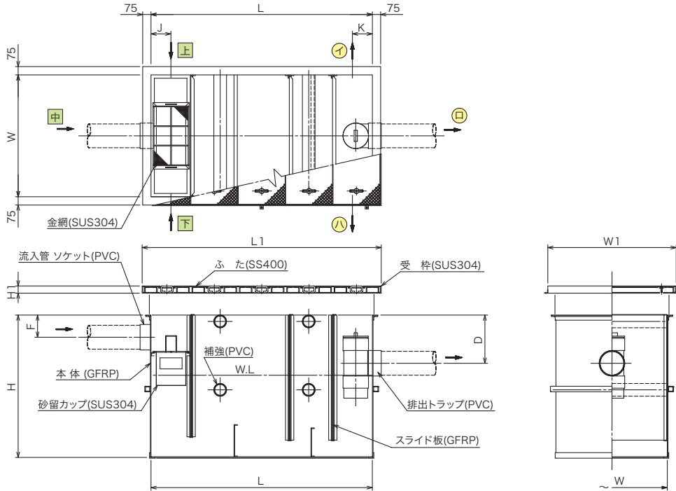
構造図
