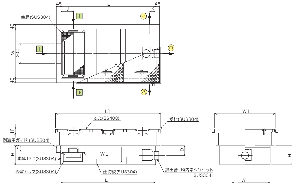
構造図
