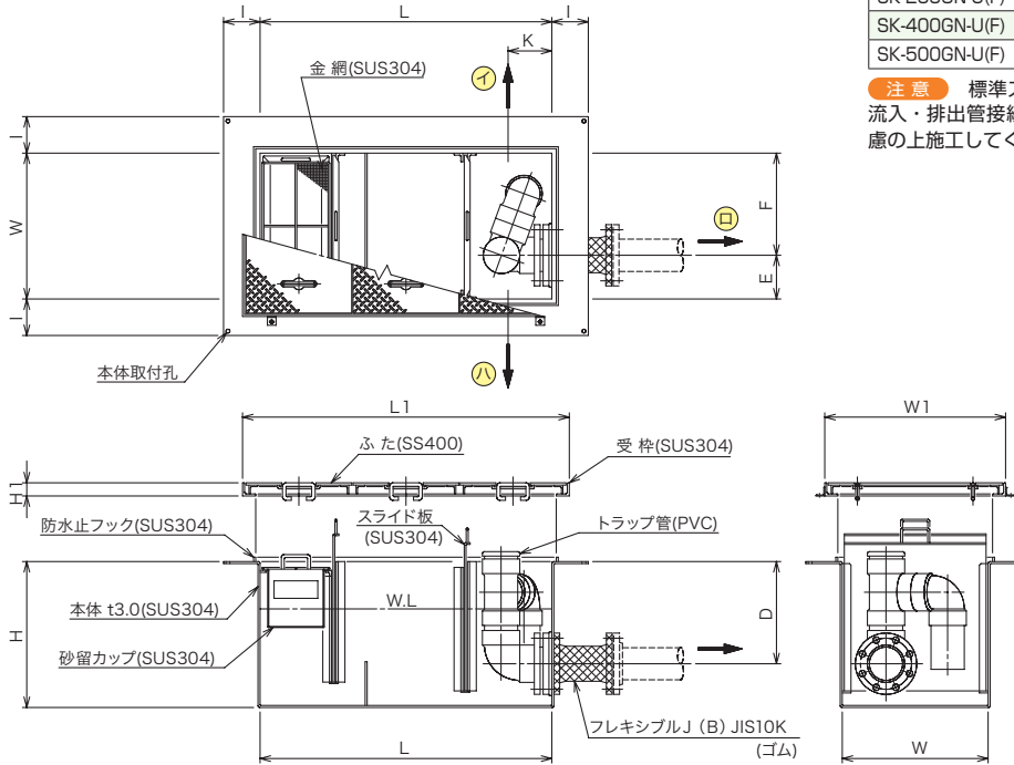
構造図
