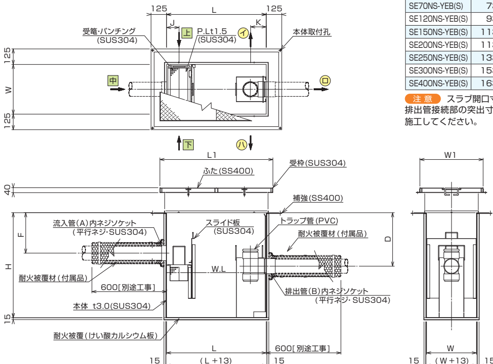
構造図
