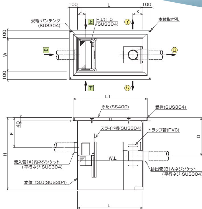
構造図
